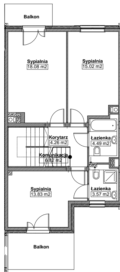
1 RZUT_PIĘTRA
