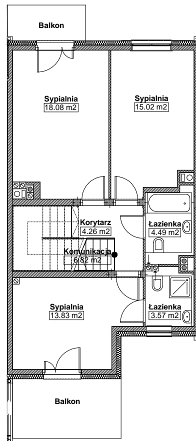
1 RZUT_PIĘTRA
